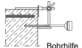
Bohrhilfe
