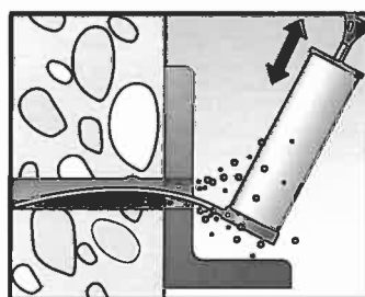
Bohrloch reinigen
