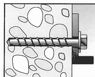
Montage Betonschraube
