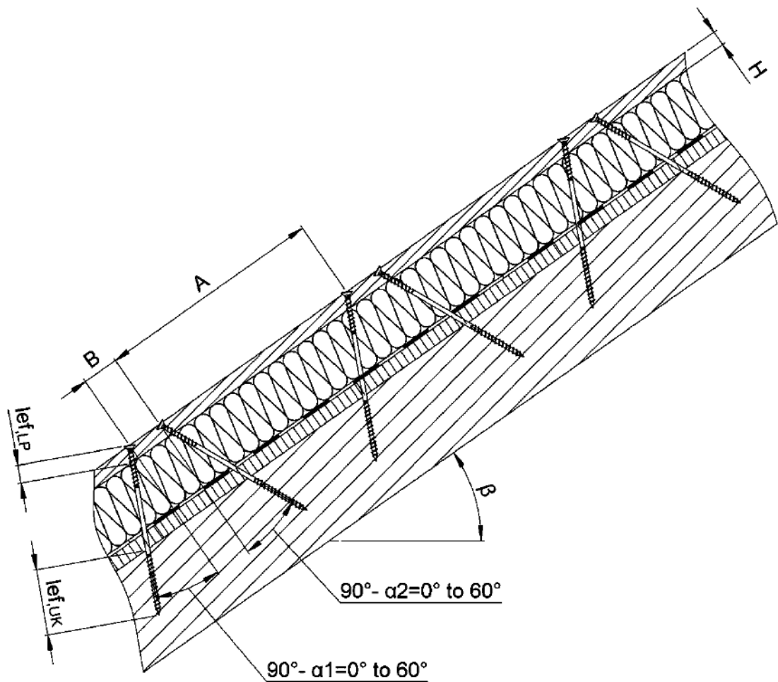
Abbildung A.4.4 Befestigung der Aufdach-Dämmung auf Sparren – Prinzipdarstellung mit wechselnder Neigung angeordneter Schrauben
