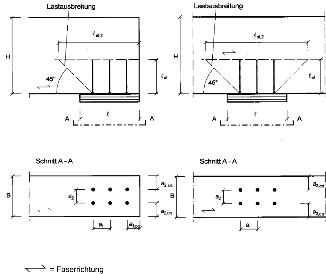
Abbildung A.3.1 Verstärktes Endauflager (links) und verstärktes Zwischenauflager (rechts)
