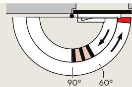
Einstellbare Öffnungsdämpfung
