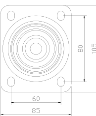
Serie LS500 Rad-Ø 100 mm
