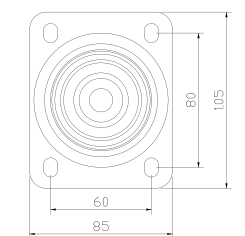
Serie LB500 Rad-Ø 100, 125 mm
