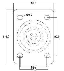
Serie LS400, LS410, LS420 ... Rad-Ø 125 mm
