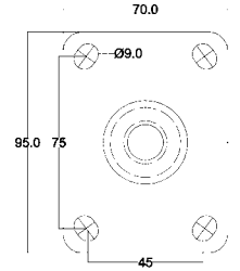
Serie C100, C110, C120 ... Rad-Ø 100, 125 mm
